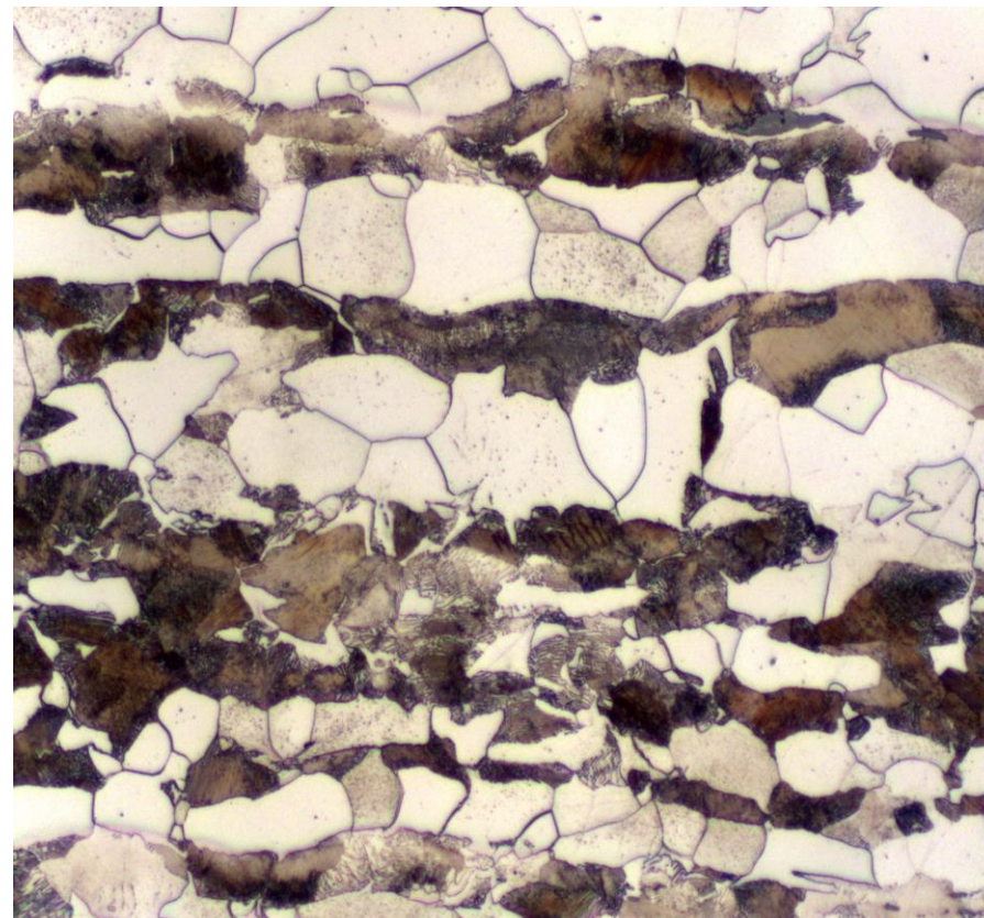
Ferritisch-perlitisches Gefüge Quelle: Eisenbeisser – Eigenes Werk
