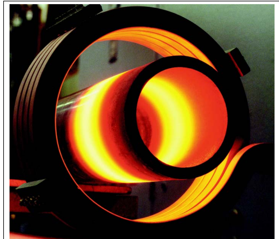
Induktive Rohrenerwärmung - SMS Elotherm, Remscheid Inductive heating of tube ends - SMS Elotherm, Remscheid, Germany
